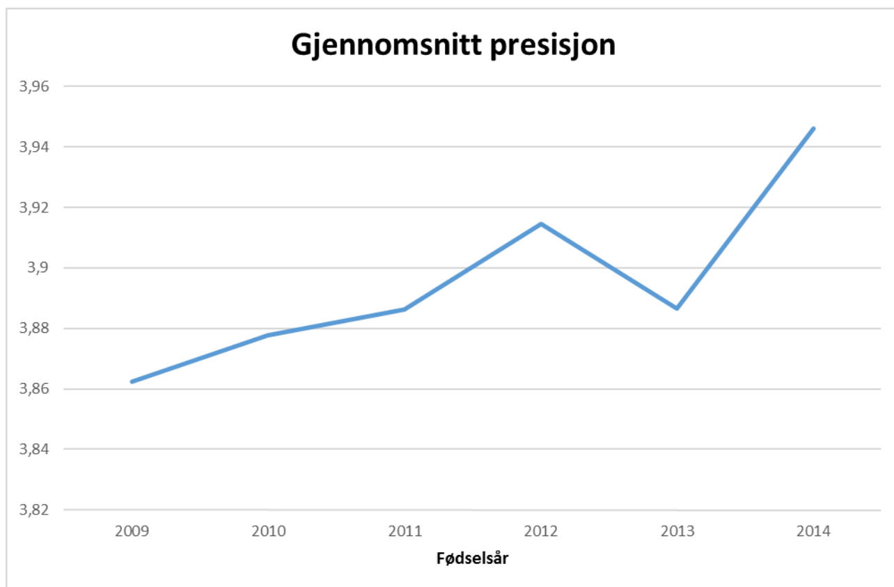
Fig. 14 – Gjennomsnittlig presisjon
